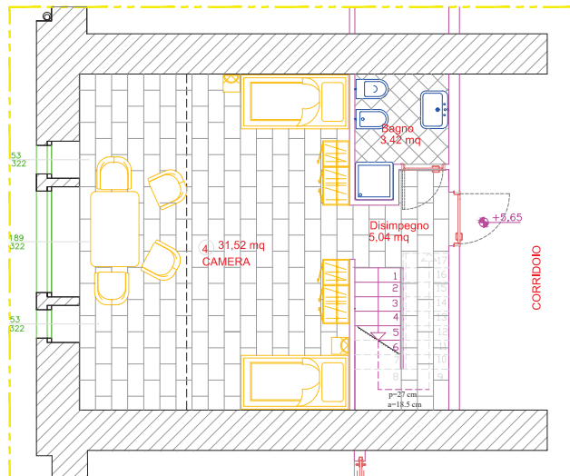
CAMERA TIPO
